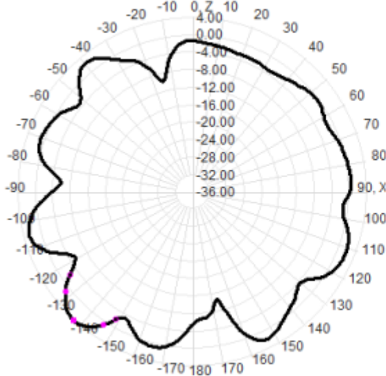
2310.0MHz Total(E1-XZ), Max= 4.00dBi
