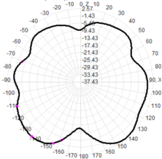
900.0MHz Total(E1-XZ), Max= 2.57dBi
