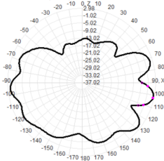
1810.0MHz Total(E1-XZ), Max= 2.12dBi
