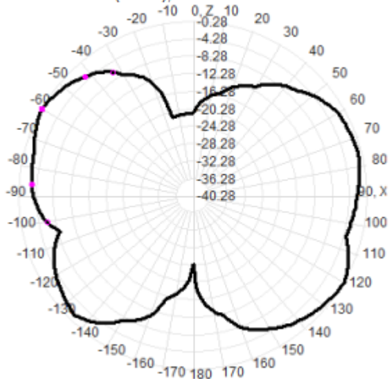
2710.0MHz Total(E1-XZ), Max=-0.28dBi
