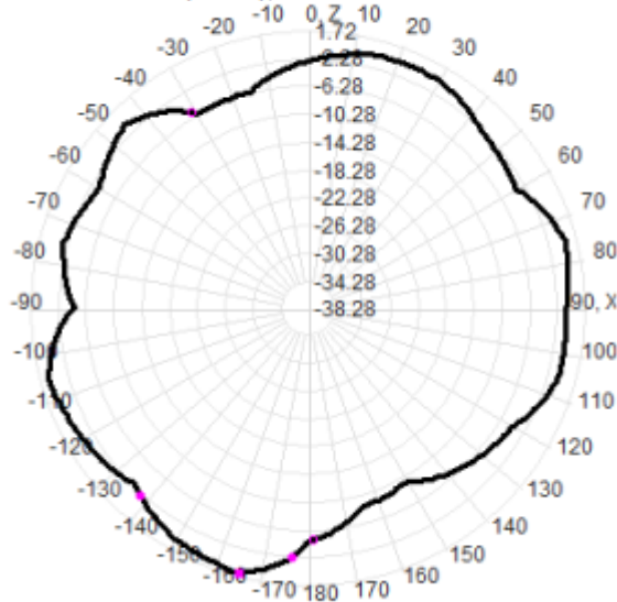
1710.0MHz Total(E1-XZ), Max= 0.90dBi
