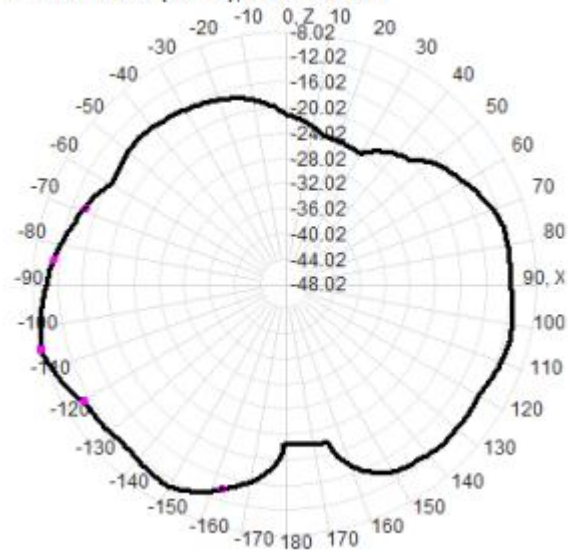
700.0MHz Total(E1-XZ), Max=-8.02dBi
