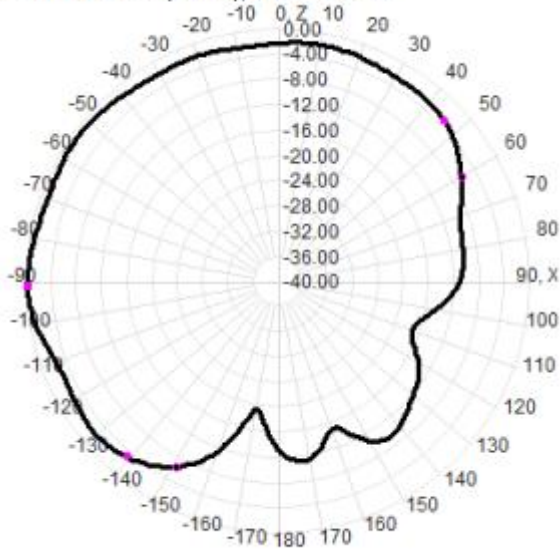
2710.0MHz Total(E1-XZ), Max= -0.33dBi
