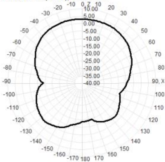
780.0MHz Total(E1-XZ), Max= 3.05dBi
