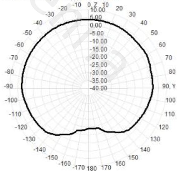
750.0MHz Total(E2-YZ), Max= 3.77dBi
