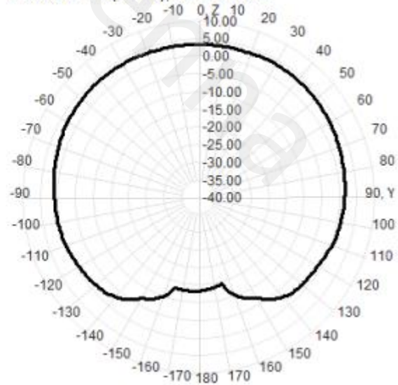
780.0MHz Total(E2-YZ), Max= 3.57dBi
