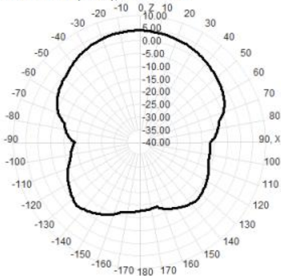
750.0MHz Total(E1-XZ), Max= 4.18dBi
